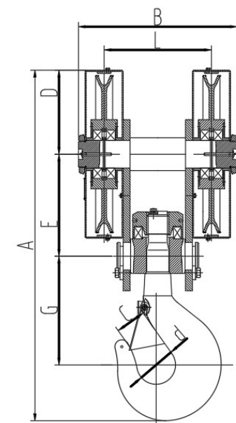
20t 吊钩组
